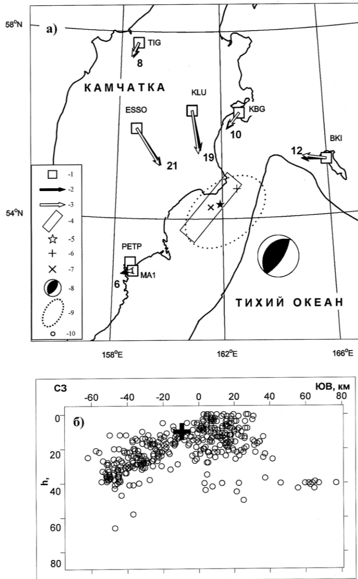
Рис. 14. Результаты восстановления характеристик статического очага Кроноцкого землетрясения по косейсмическим смещениям (горизонтальные компоненты), зарегистрированным GPS-станциями: положение статического очага и вектора горизонтальных смещений относительно станции "Петропавловск Камчатский" (а); проекции на вертикальную плоскость, ориентированную вкост фокальной зоны, гипоцентров афтершоков за период 5-31 декабря, в определении координат которых обязательно участвовали фазы Р- и S-волн на ближайшей к очагу станции (б).
