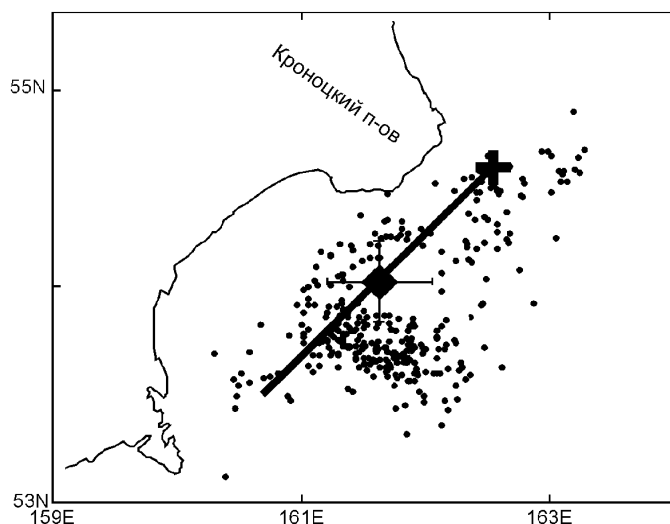
Рис. 7. Результаты восстановления пространственных характеристик высокочастотного (0.5-2.0 Гц) очага Кроноцкого землетрясения по телесейсмическим записям Р-волн
