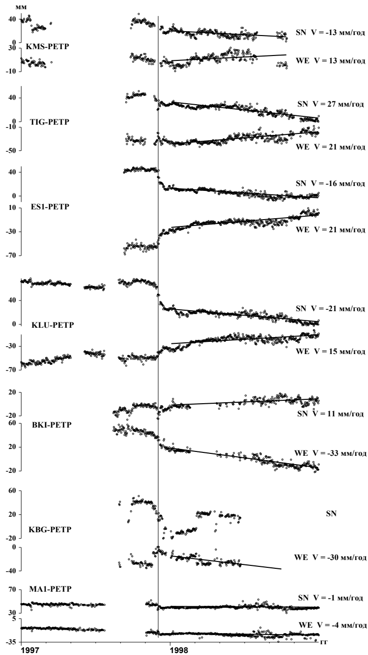
Рис. 13. Смещения пунктов относительно станции "Петропавловск-Камчатский" по направлениям север-юг (NS) и запад-восток (WE)
