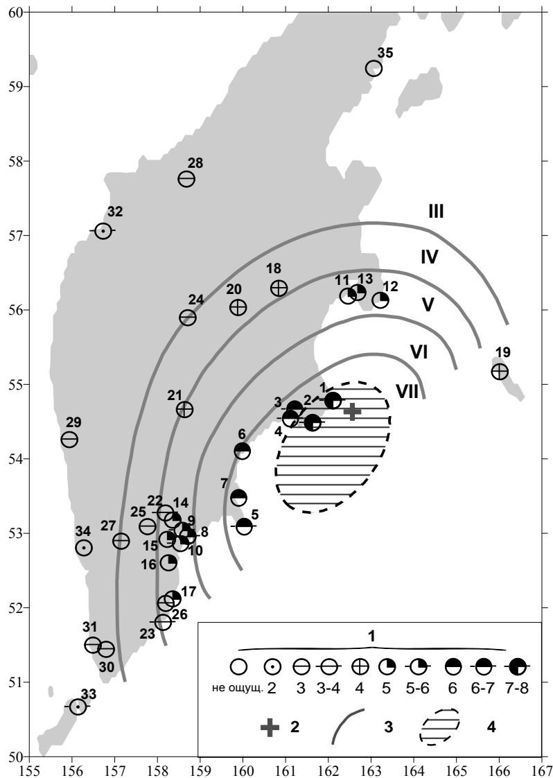
Рис. 9. Карта изосейст Кроноцкого землетрясения 05.12.1997 г. в 11^{\text{h}}26^{\text{m}} с M_w=7.8
