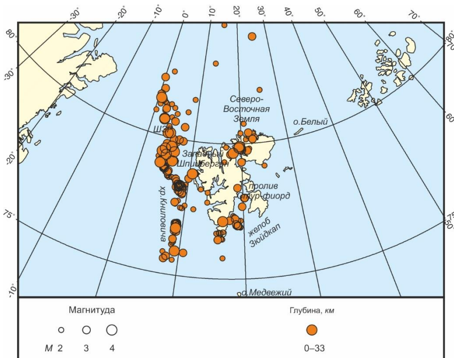
Рис. III.17. Карта эпицентров землетрясений с M_L \geq 2 в районе архипелага Шпицберген и прилегающей акватории в 2019 г.
