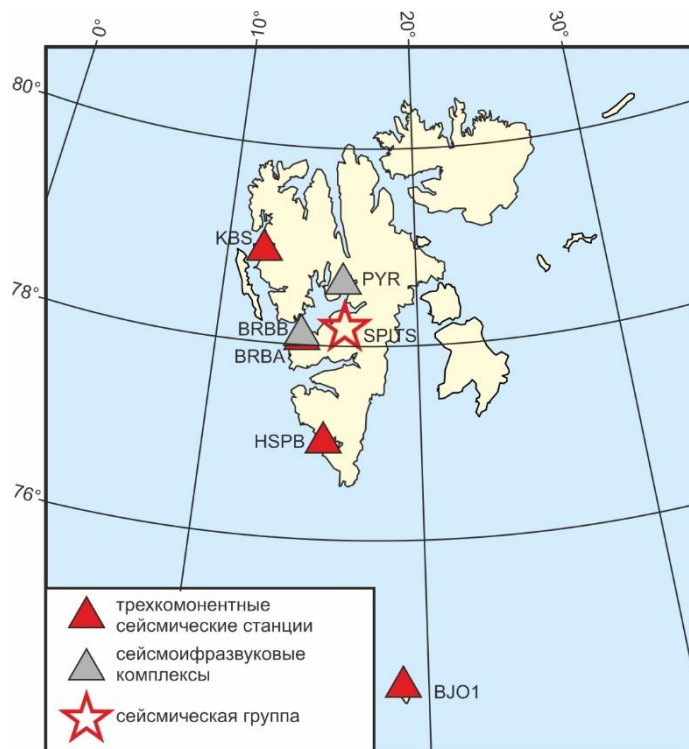
Рис. III.16. Международная сеть сейсмических и сейсмоинфразвуковых станций в районе архипелага Шпицберген в 2019 г.
