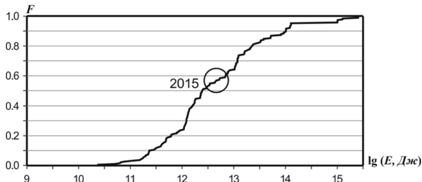
Рис. II.10. Функция распределения сейсмической энергии для региона Северо-Восток России и Чукотка
