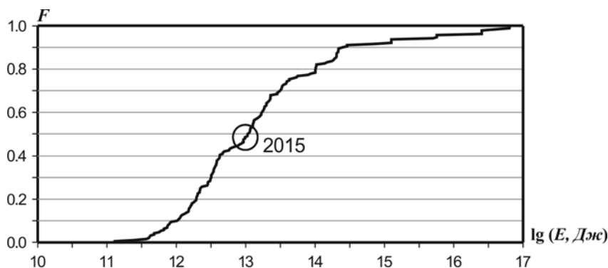
Рис. II.9. Функция распределения сейсмической энергии для региона Якутия
