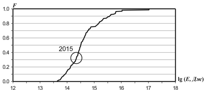
Рис. II.11. Функция распределения сейсмической энергии для региона Камчатка и Командорские острова
