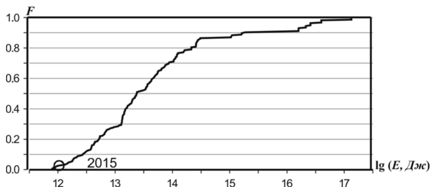
Рис. II.4. Функция распределения сейсмической энергии для региона Алтай и Саяны
