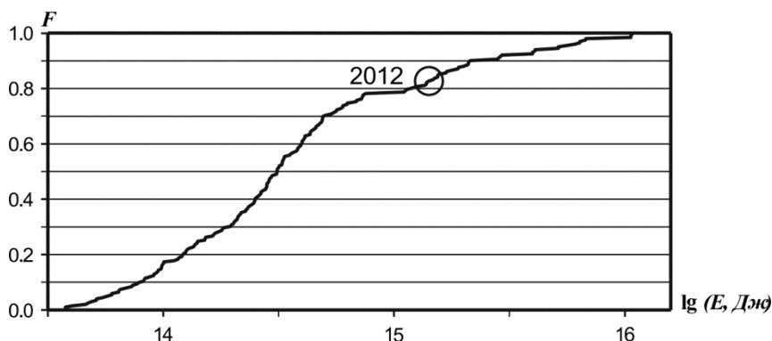
Рис. II.11. Функция распределения сейсмической энергии для региона Камчатка и Командорских островов
