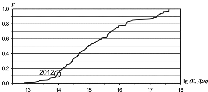
Рис. П.8. Функция распределения сейсмической энергии для Курило-Охотского региона
