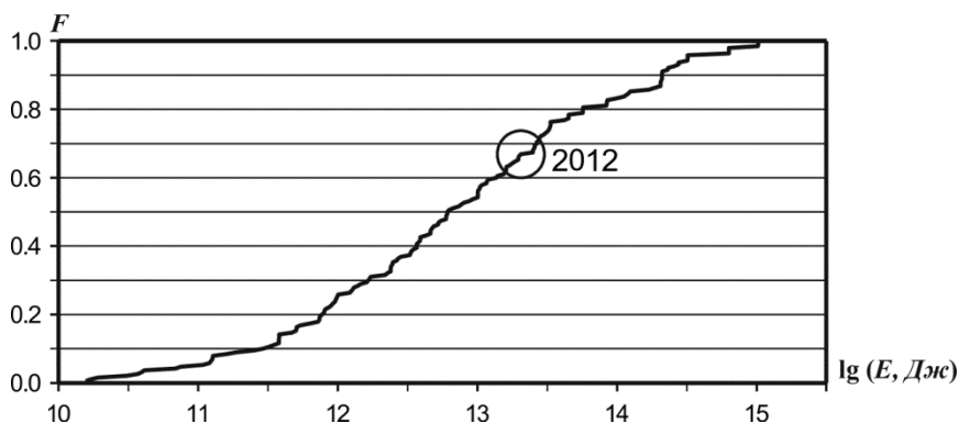
Рис. П.3. Функция распределения сейсмической энергии для региона Арктика
