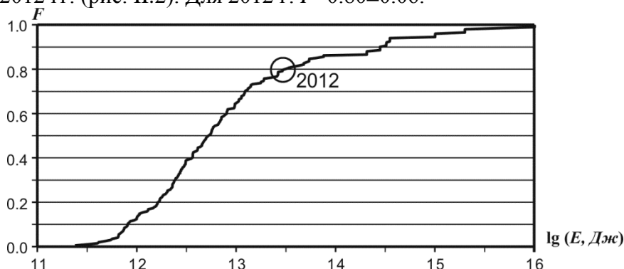
Рис. П.2. Функция распределения сейсмической энергии для региона Северный Кавказ
