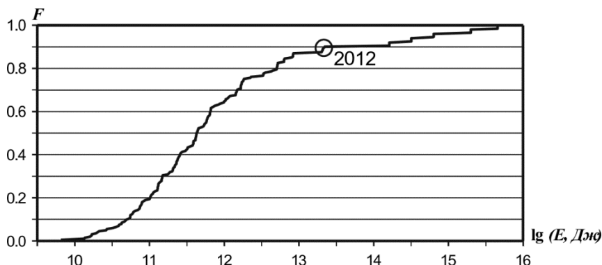
Рис. П.7. Функция распределения сейсмической энергии для региона Сахалин
