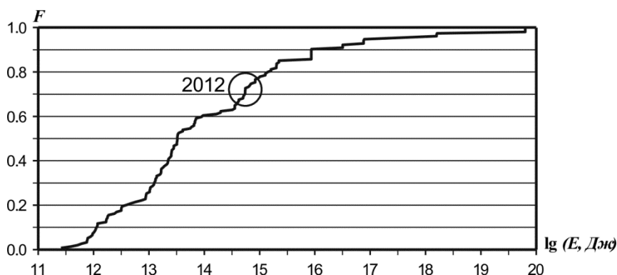
Рис. П.6. Функция распределения сейсмической энергии для региона Приамурье и Приморье
