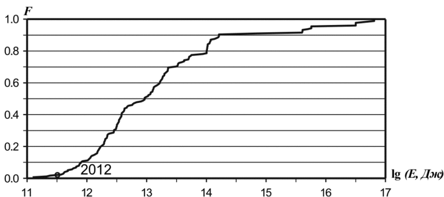
Рис. П.9. Функция распределения сейсмической энергии для Якутского региона
