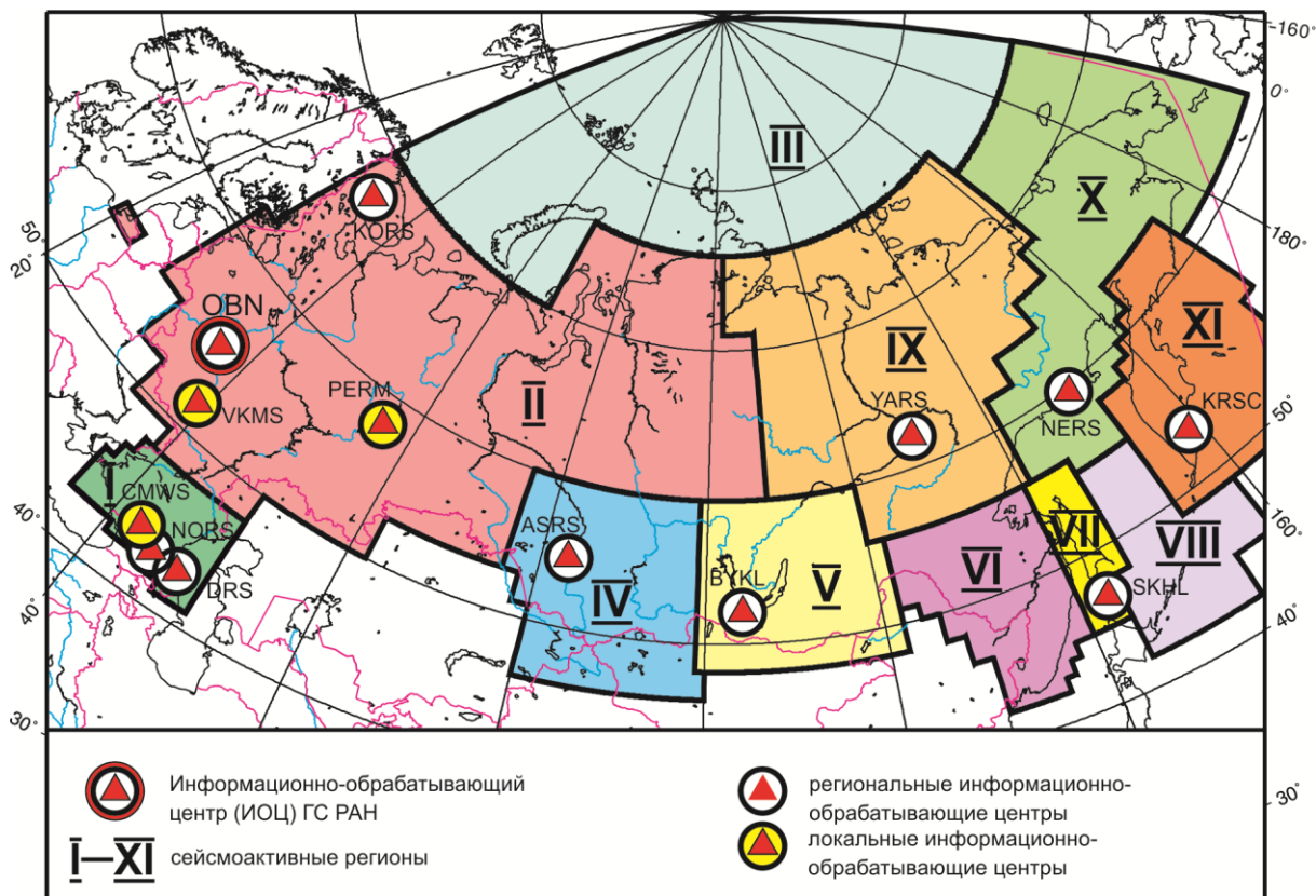
Рис. II.1. Границы регионов на территории России
