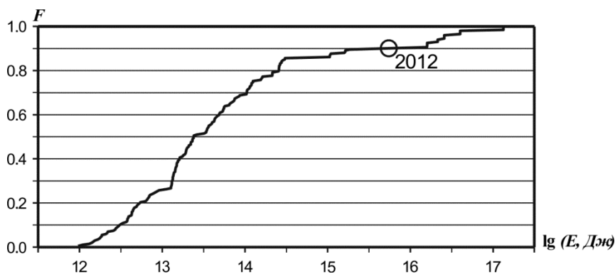
Рис. П.4. Функция распределения сейсмической энергии для региона Алтай и Саяны
