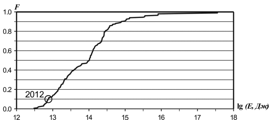
Рис. П.5. Функция распределения сейсмической энергии для региона Прибайкалье и Забайкалье
