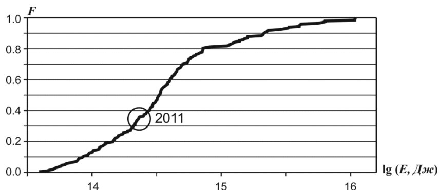
Рис. II.11. Функция распределения сейсмической энергии для региона Камчатка и Командорских островов
