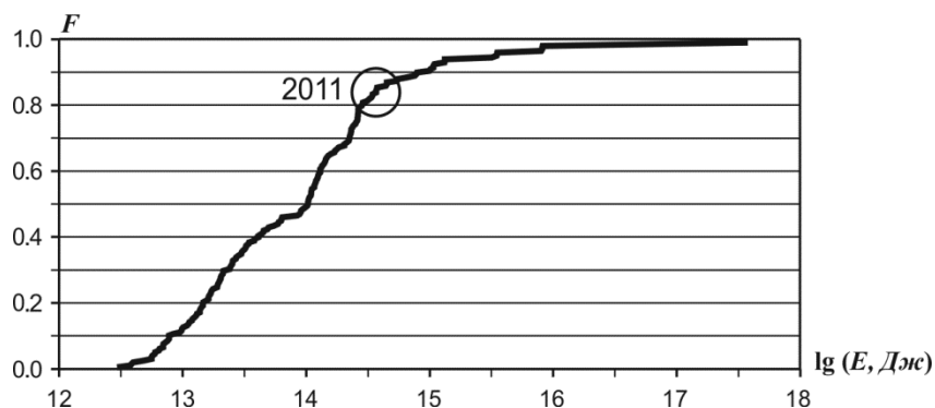
Рис. II.5. Функция распределения сейсмической энергии для региона Прибайкалье и Забайкалье
