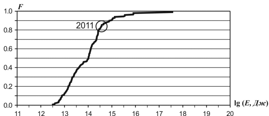
Рис. II.6. Функция распределения сейсмической энергии для региона Приамурье и Приморье
