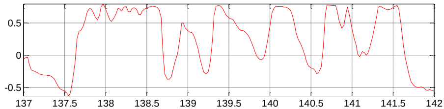
Рис. 9. График поперечного сечения коррелограммы в полосе 137.7–138.7 с
