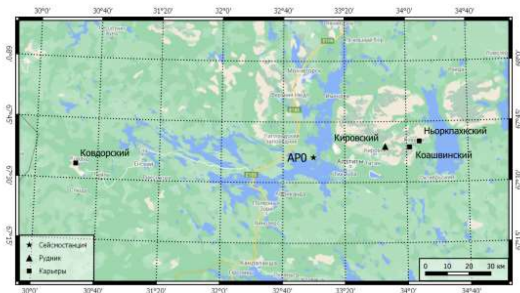
Рис. 1. Обзорная карта расположения горных выработок, в которых производились взрывы, зарегистрированные станцией АР0
