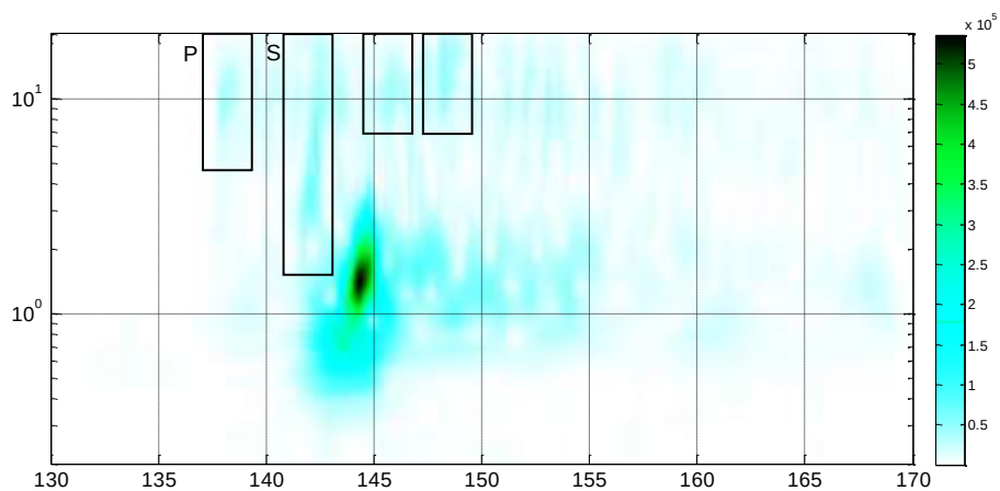
Рис. 5. Энергограмма записи взрыва № 1.
