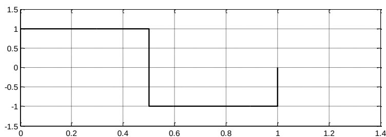
Рис. 10. Вейвлет Хаара
