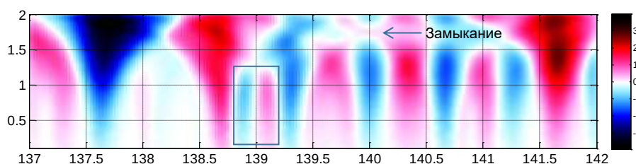
Рис. 11. Хаарограмма значений поперечного сечения коррелограммы.
