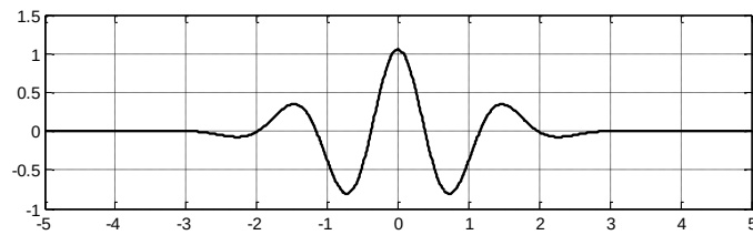
Рис. 3. Вейвлет Гаусса 8-го порядка
