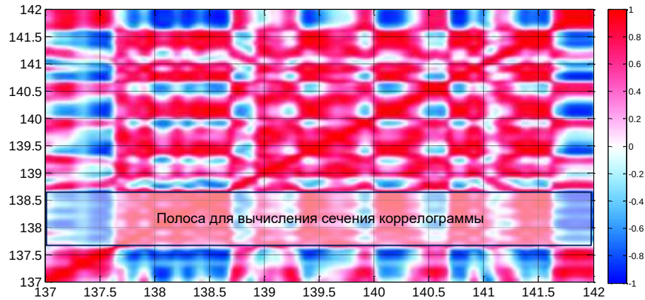
Рис. 8. Коррелограмма фрагмента записи продольных волн.
