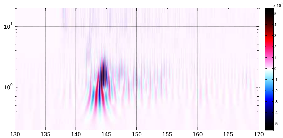
Рис. 4. Вейвлетограмма записи взрыва № 1.
