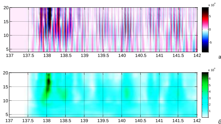
Рис. 7. Вейвлетограмма и энергограмма фрагмента записи продольных волн: а – вейвлетограмма в высокочастотной части спектра; б – энергограмма по вейвлетограмме
