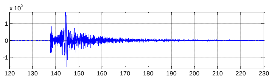
Рис. 2. Запись Z-канала станции АР0 для взрыва № 1.
