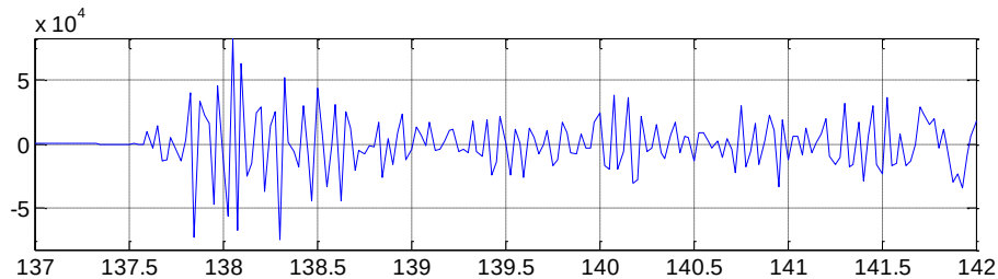
Рис. 6. Фрагмент записи до вступления поперечной волны.
