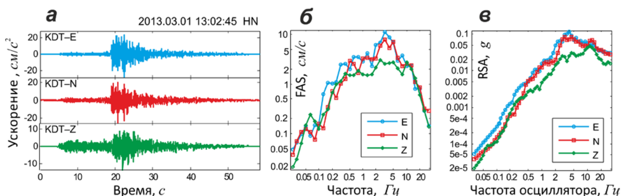
Рис. 8. Три компоненты записи ускорения грунта от землетрясения 1 марта в 13 h 20 m (а), сглаженные амплитудные спектры Фурье (FAS) (б) и спектры реакции по ускорению (RSA) (в) для этих записей.
