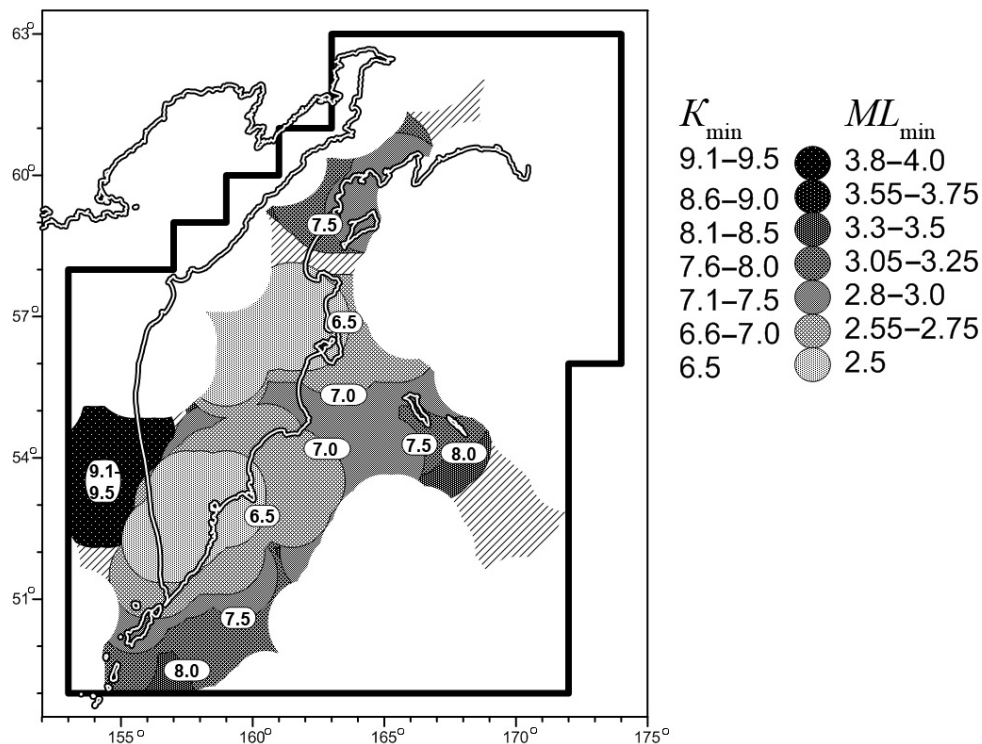
Рис. 2. Карта региональной представительности каталога землетрясений 2013 г. в зоне ответственности КФ ФИЦ ЕГС РАН.
