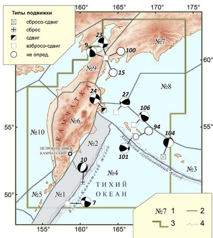
Рис. 7. Карта эпицентров и стереограммы механизмов очагов сильных землетрясений ( K_S \geq 11.6 ) зон № 3–10 за 2013 г.
