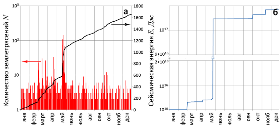
Рис. 5. Гистограмма распределения и кумулятивный график суточного числа землетрясений с K_S \geq 8.6 (а); кумулятивный график выделившейся сейсмической энергии \Sigma E (б) в 2013 г. для зоны ответственности сети КФ ФИЦ ЕГС РАН
