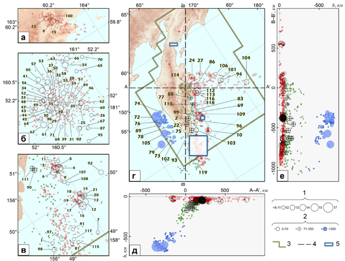
Рис. 3. Карта эпицентров землетрясений Камчатки с K_S \geq 8.6 за 2013 г. (г) и расширенная карта сейсмичности в районах Камчатского перешейка (а), Тихого океана напротив Авачинского залива (б) и вблизи северных Курил (в); проекции на вертикальные плоскости А–А' (д) и В–В' (е).
