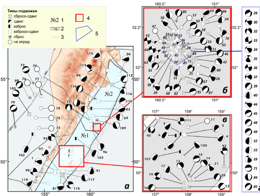
Рис. 6. Карта эпицентров и стереограммы механизмов очагов сильных землетрясений ( M_s \geq 11.6 ) Курило-Камчатской зоны субдукции (зоны № 1 и 2) за 2013 г. (а) и расширенная карта сейсмичности в районе Тихого океана напротив Авачинского залива (б) и вблизи Северных Курил (в).
