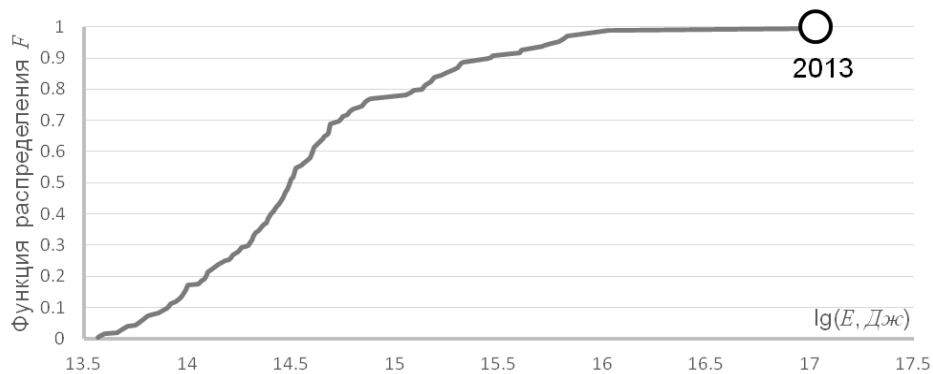
Рис. 4. Функция распределения F сейсмической энергии для региона Камчатки и Командорских островов.
